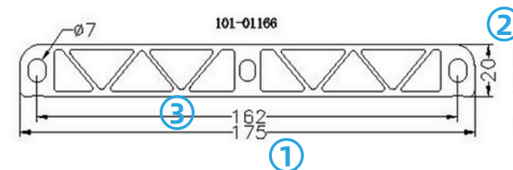
バッテリーエンドプレートA
