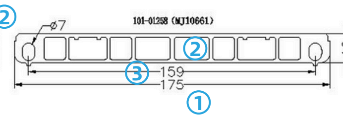
バッテリーエンドプレートB
